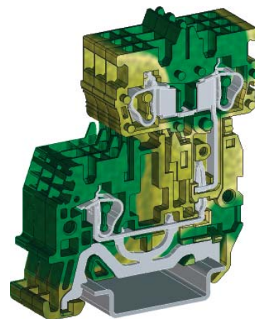
Пример установки CHTE.2D
