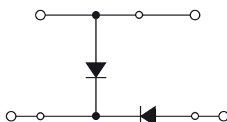
Электрическая схема
